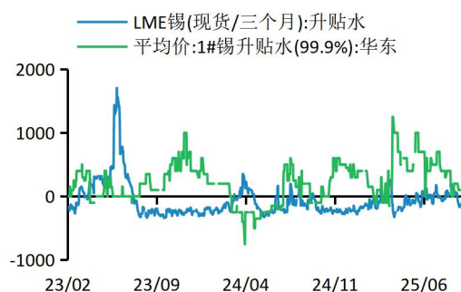
图2 锡现货基差
