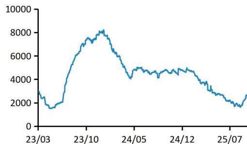
图 10 LME 锡库存
