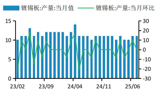
图5 镀锡板产量
