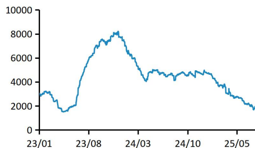
图 6 LME 锡库存
