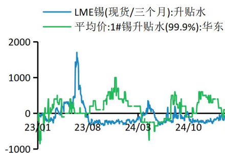
图 3 锡现货基差
