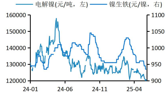
图2 镍现货价格走势
